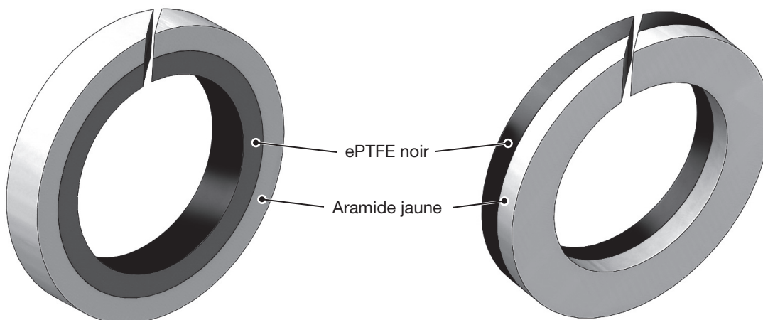
Figure 1 – Bague d'étanchéité principale (REPRESENTEE AVEC L'ETANCHEITE DE L'ARBRE REALISEE PAR DE L'ePTFE NOIR)
